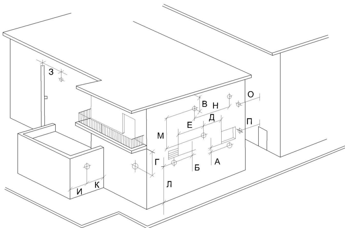
Рисунок 1 – Размещение отверстий дымоходов от теплогенераторов и водонагревателей с закрытой камерой сгорания на фасаде жилого дома
