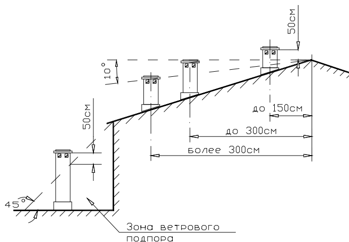
Рисунок 3 – Расположение дымоходов с учетом зоны ветрового подпора
