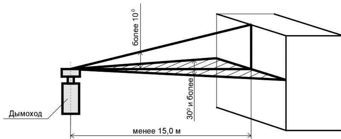
Рисунок 4 – Расположение дымохода относительно соседнего объекта
